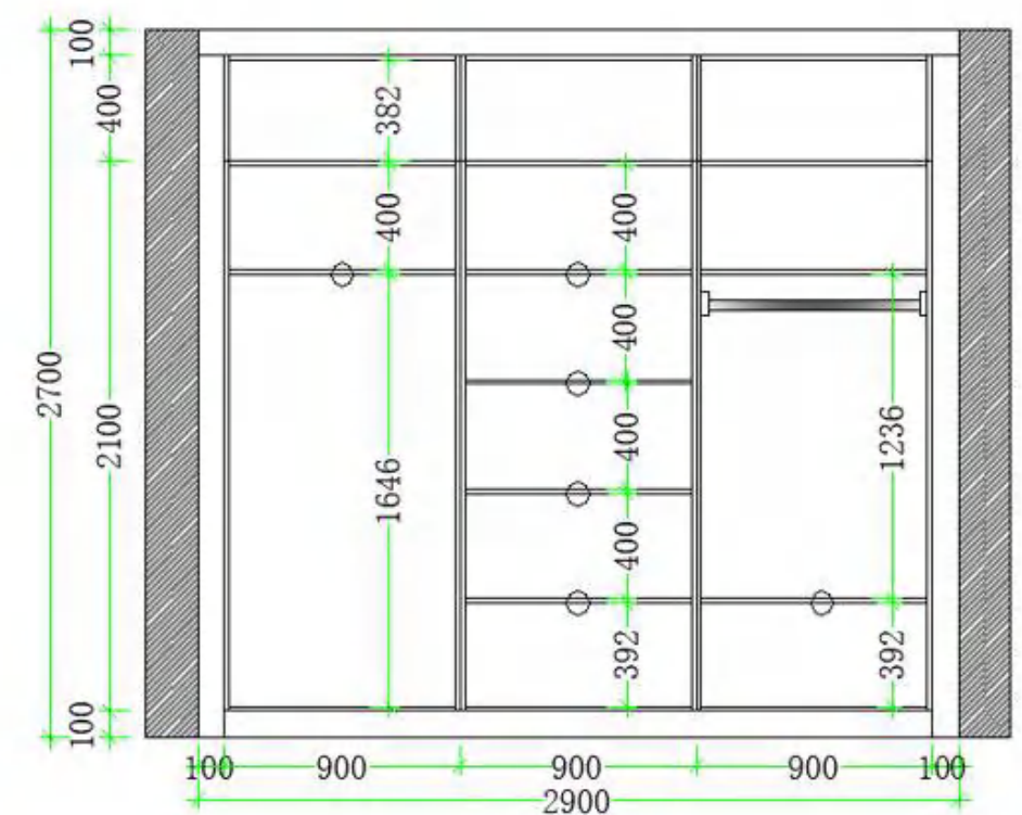
ELEVATION A
