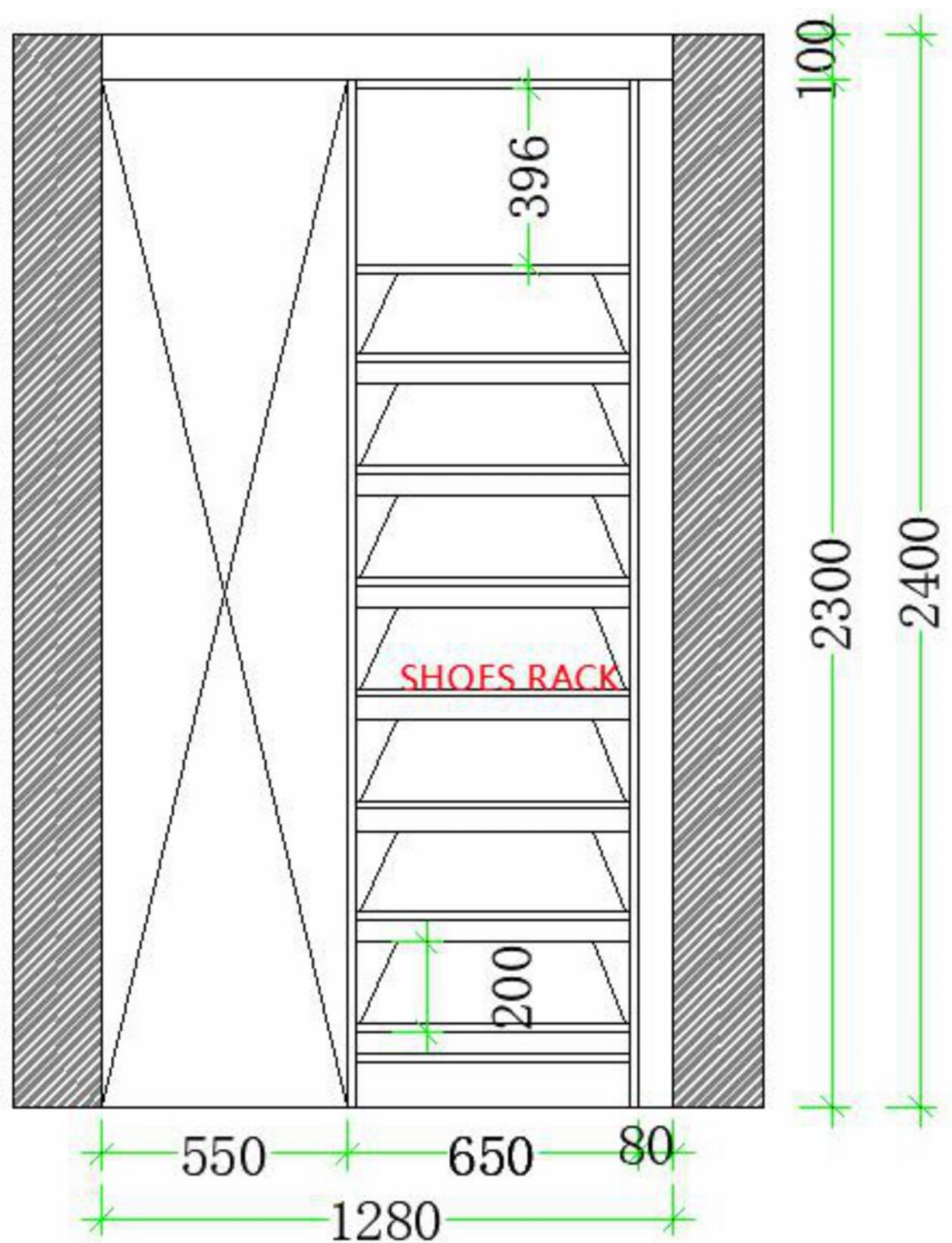
ELEVATION E
