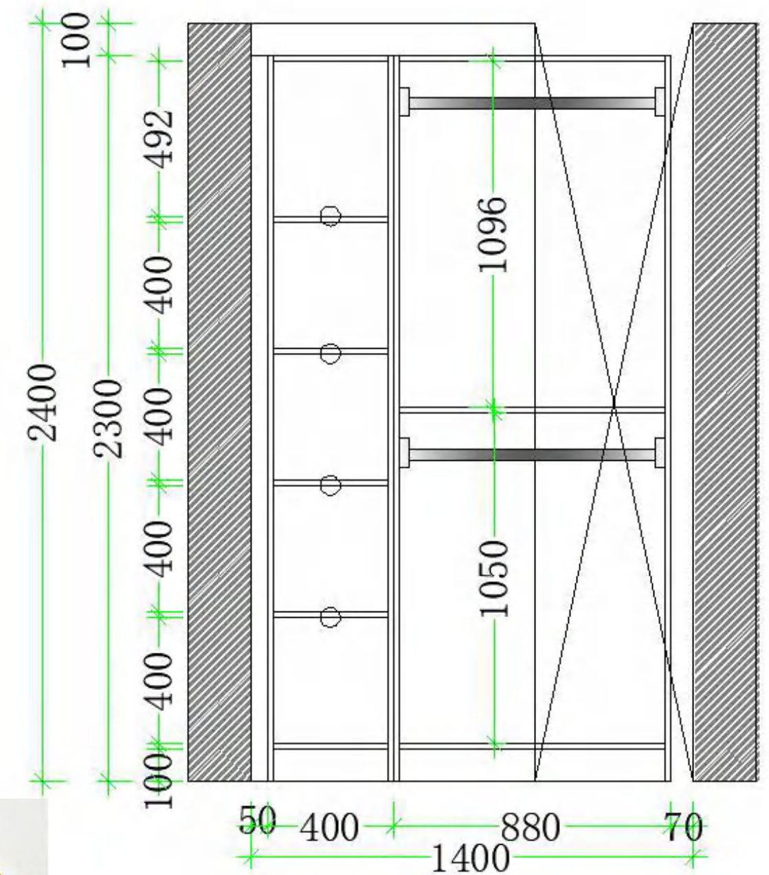
ELEVATION A
