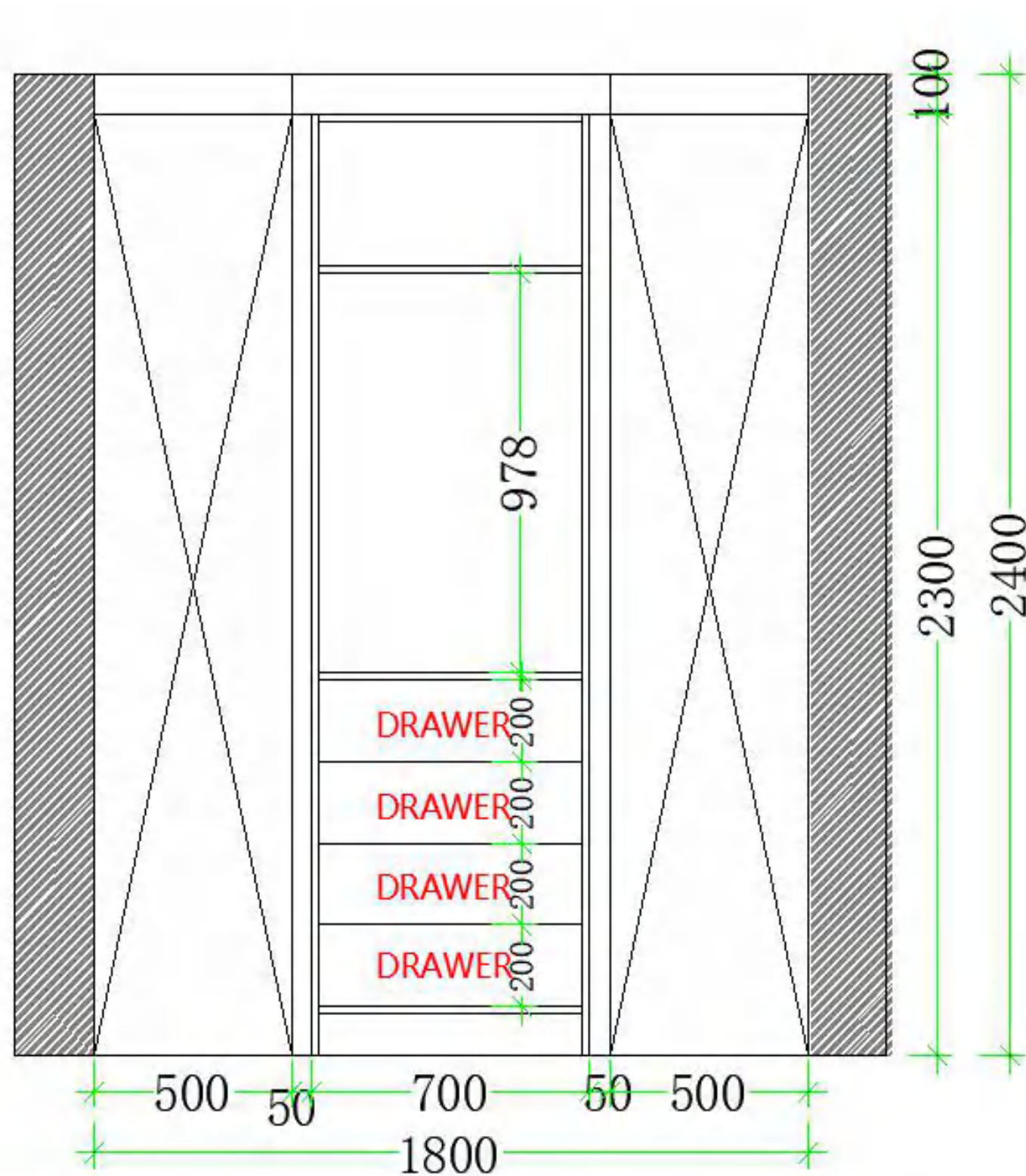
ELEVATION B
