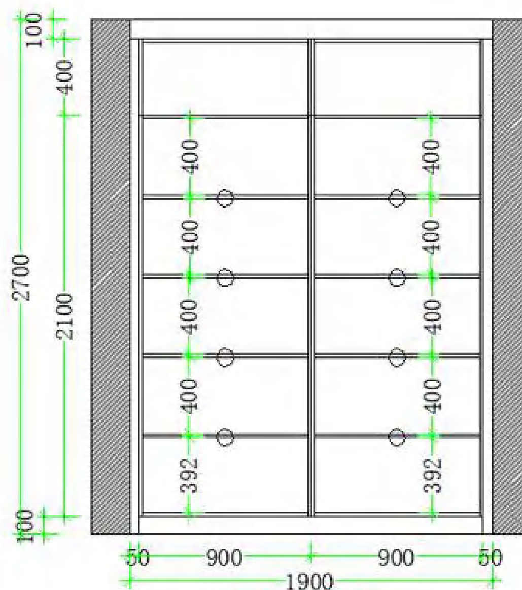
ELEVATION A
