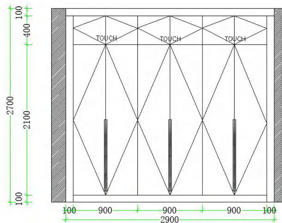
ELEVATION A
