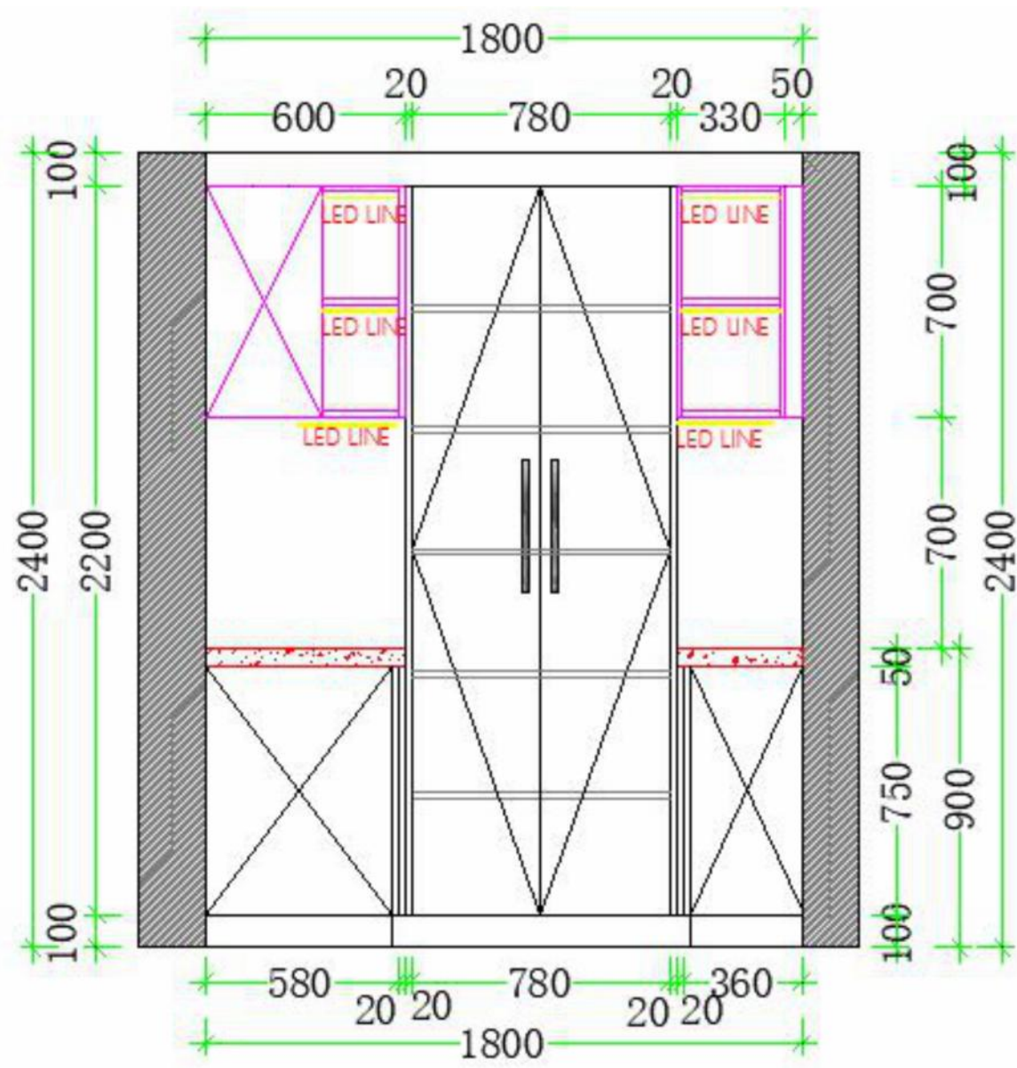
ELEVATION B
